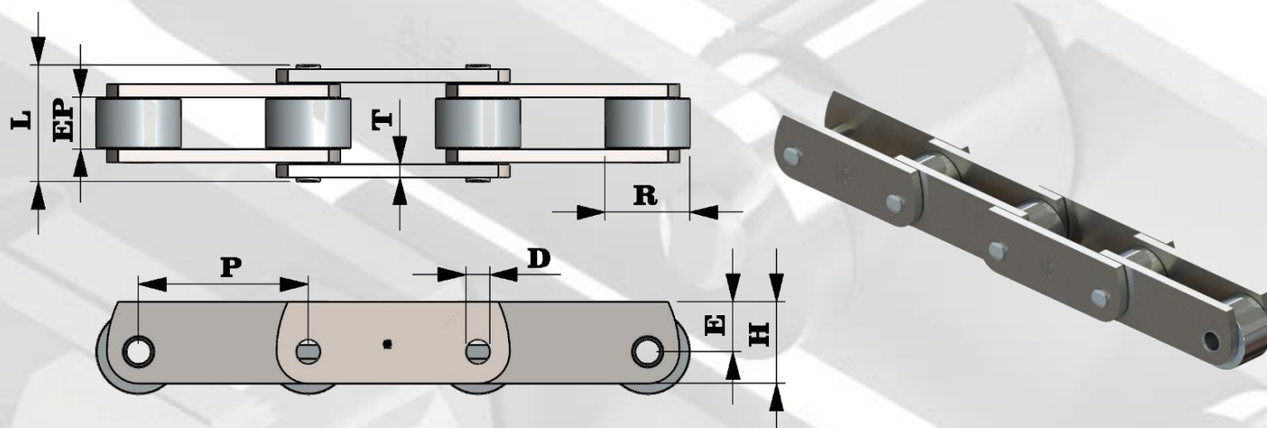
CORRENTE TRANSPORTADORA - PINO SÓLIDO PLACA ALTA ( PSPA )
