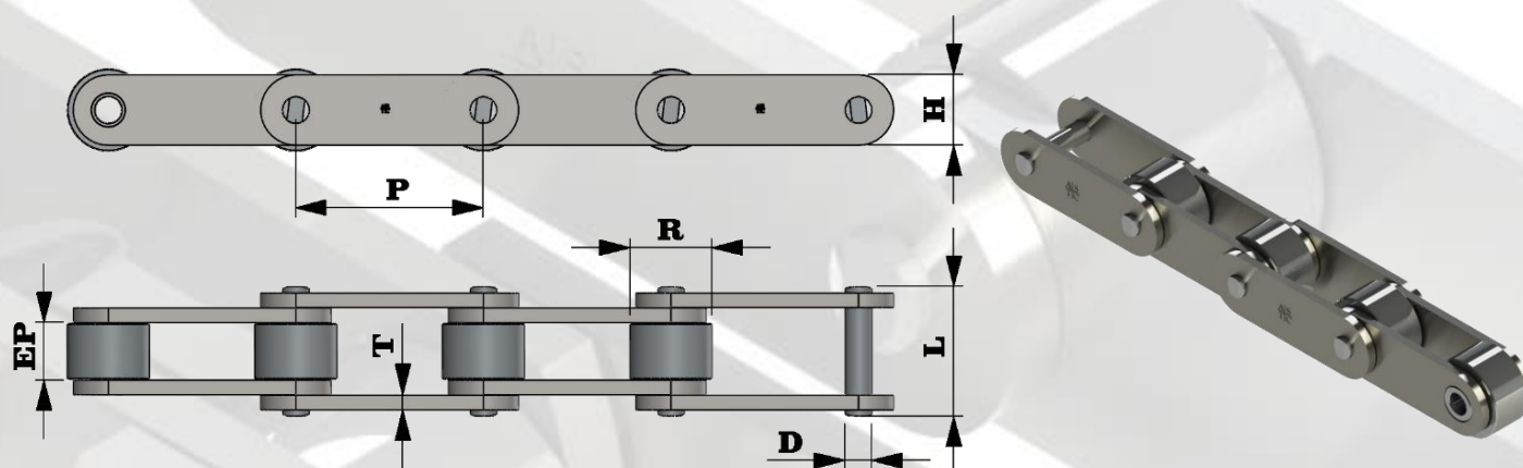
CORRENTE TRANSPORTADORA - PINO SÓLIDO ROLO GRANDE ( PSRG )
