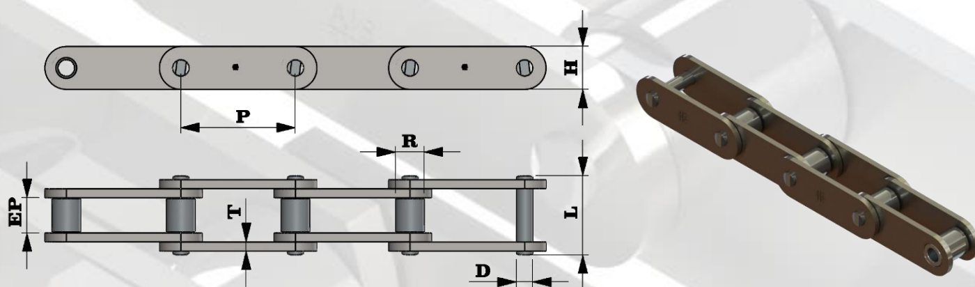
CORRENTE TRANSPORTADORA - PINO SÓLIDO ROLO PEQUENO (PSRP)
