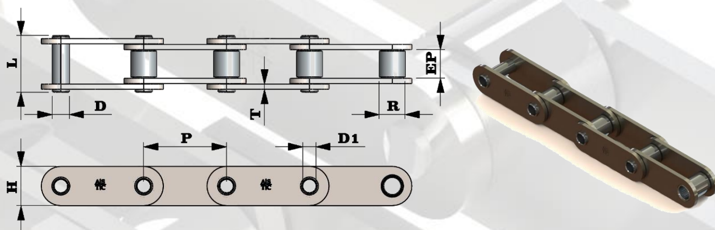
CORRENTE TRANSPORTADORA - PINO OCO ROLO PEQUENO (PORP)
