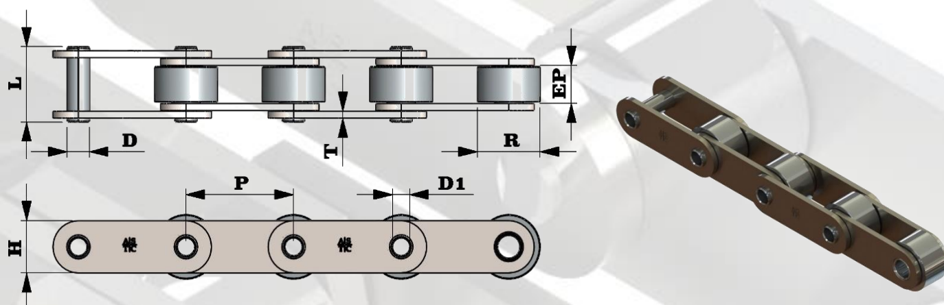
CORRENTE TRANSPORTADORA - PINO OCO ROLO GRANDE ( PORG )
