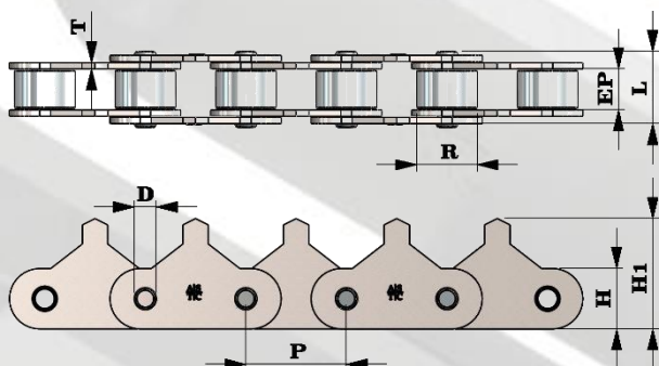
CORRENTE PASSO LONGO ADICIONAL A-1 e K-1
