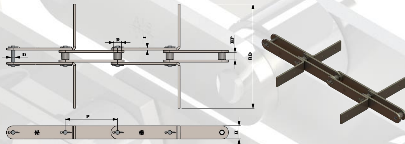
CORRENTE TRANSPORTADORA - TIPO REDLER PARA ARRASTE (RDL)
